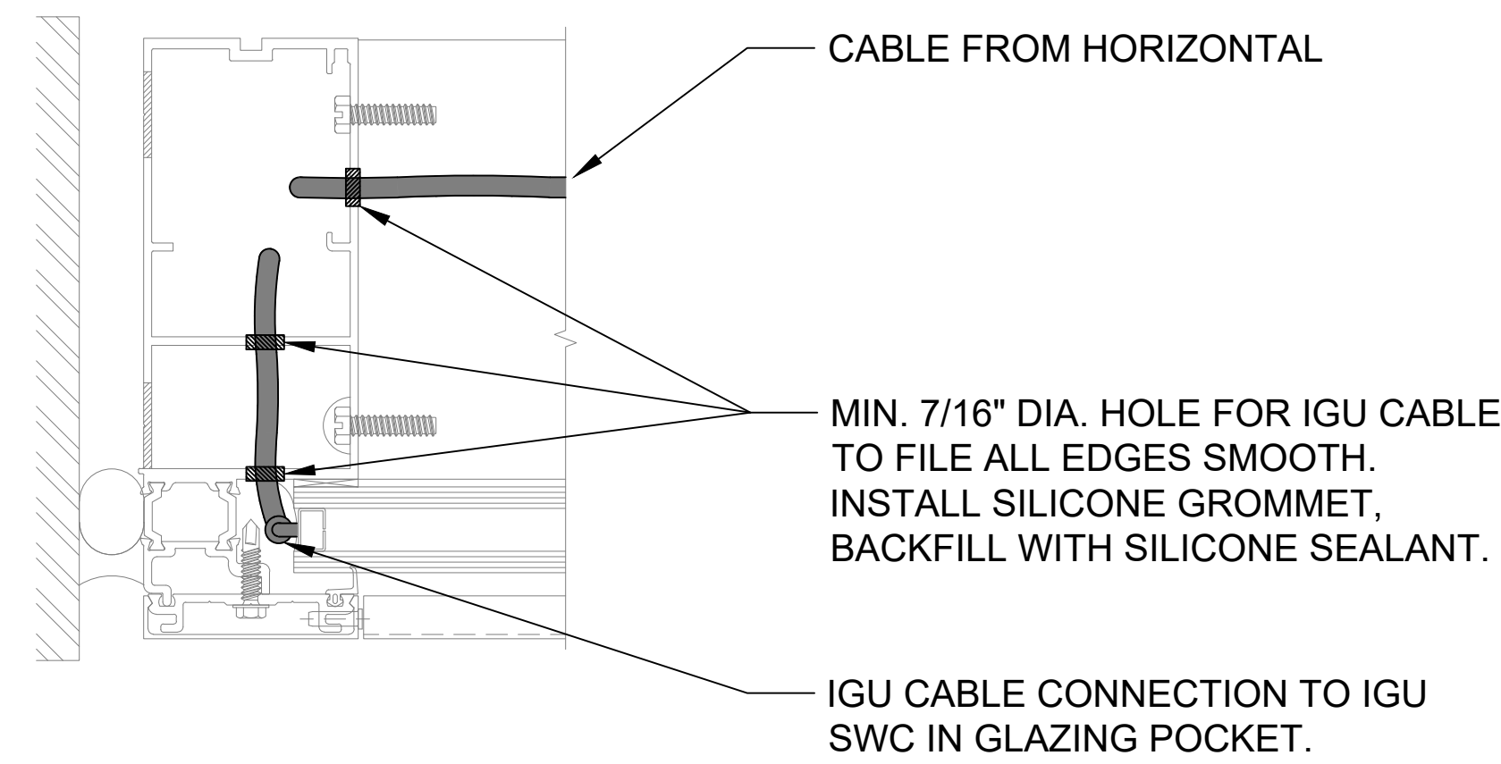
DETAIL 4 LEFT JAMB
